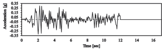
Fig. 11 El Centro NS 1940 EGM
