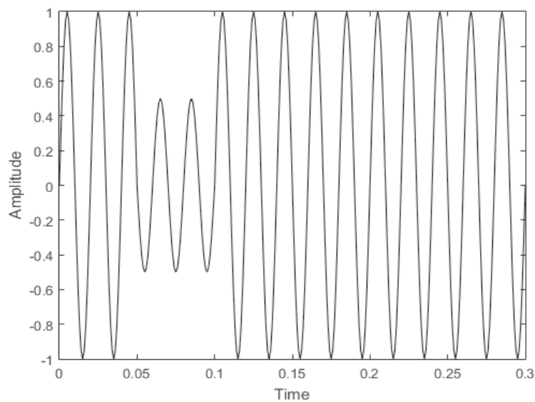
Fig. 2 Sag signal
