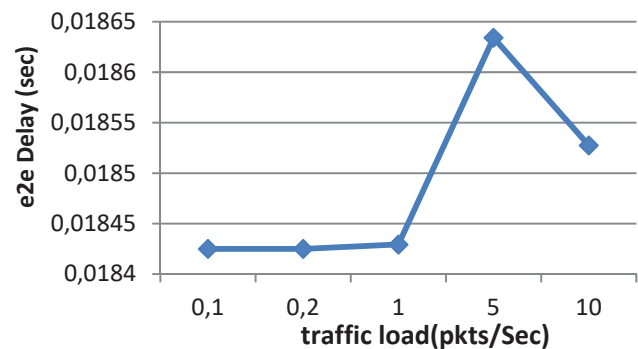
Fig. 10 E2e Delay
