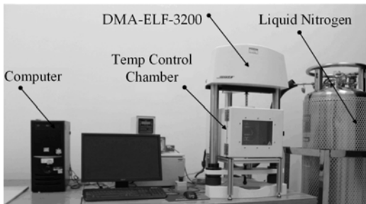
Fig. 3 DMA apparatus
