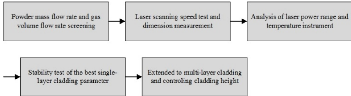
Fig. 6 Parameter testing process design
