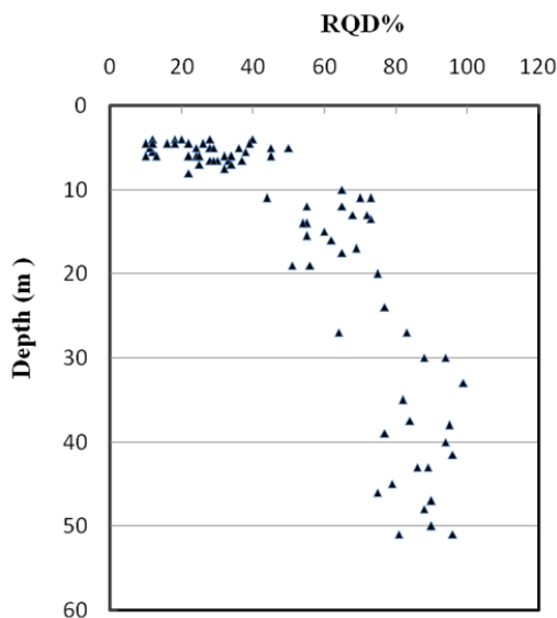
Fig. 3 RQD index values versus depth
