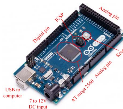
Fig. 2 Arduino mega 2560
