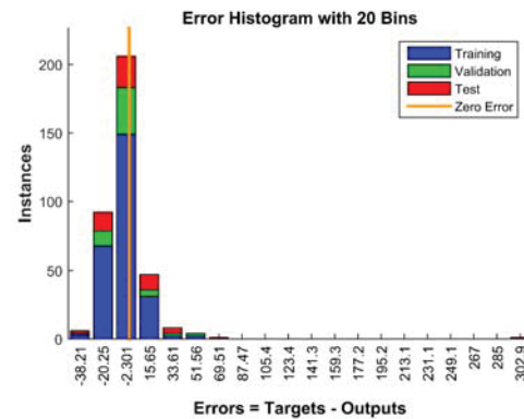
Fig. 8 Error histogram
