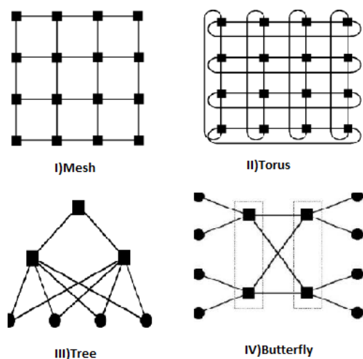
Fig. 1 NoC topologies
