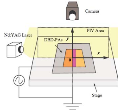
Fig. 4 PIV setup
