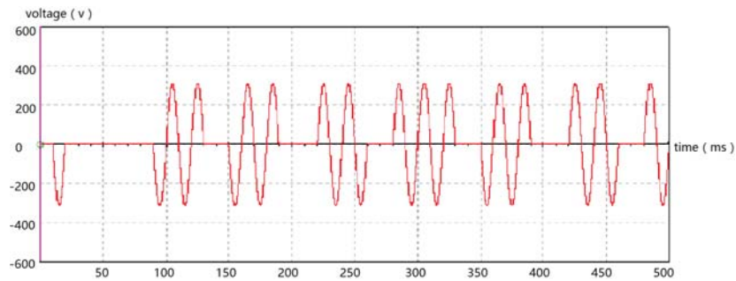
Fig. 9 Output voltage wave (d)
