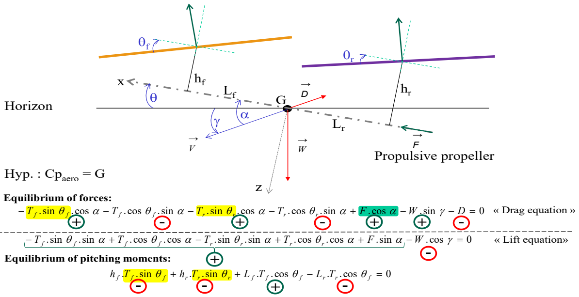
Fig. 11 Scheme of the longitudinal equilibrium
