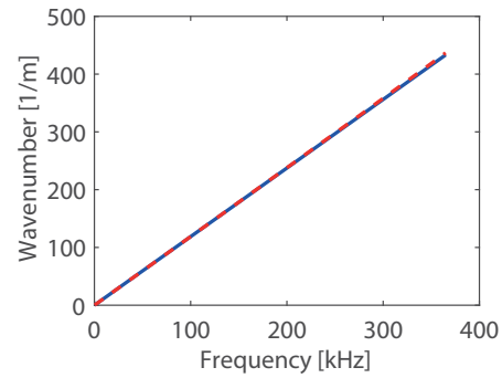
Fig. 4 Dispersion curves for the bar: Analytical(-), WFE(- -)
