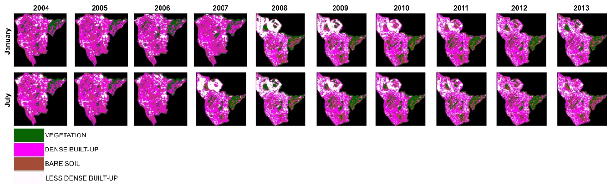
Fig. 6 Intra-urban classification using ISODATA
