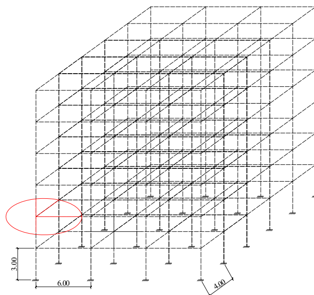
Fig. 1 Actual analyzed structure
