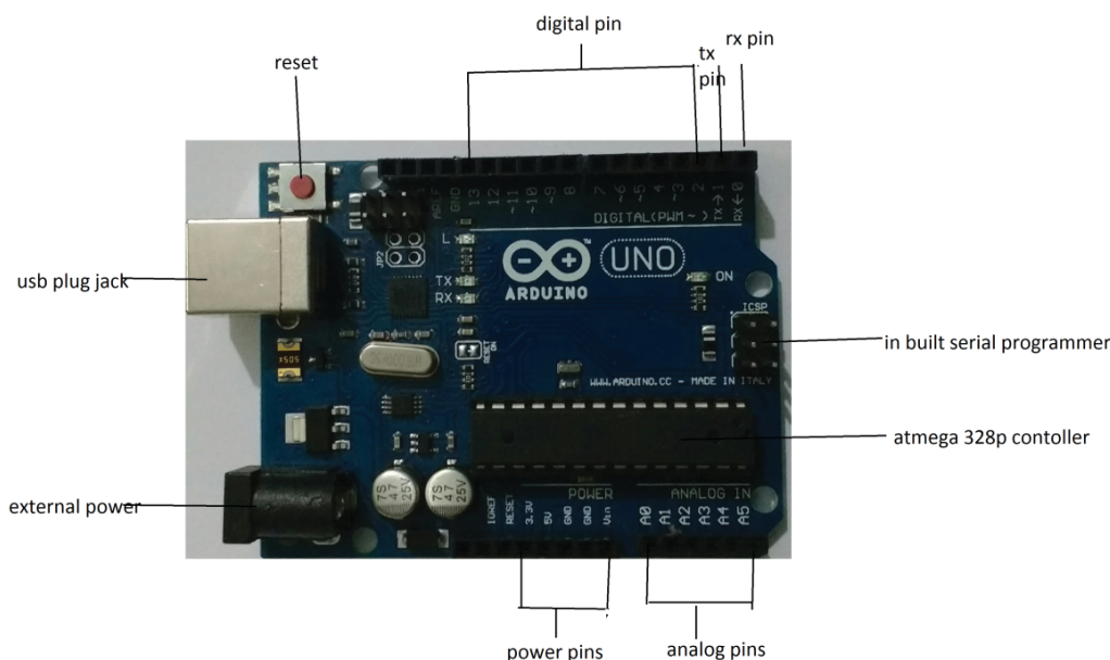
Fig. 3 Circuit of Arduino UNO
