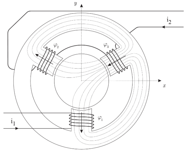
Fig. 2 Three-pole AMB with 2 coil currents [5]
