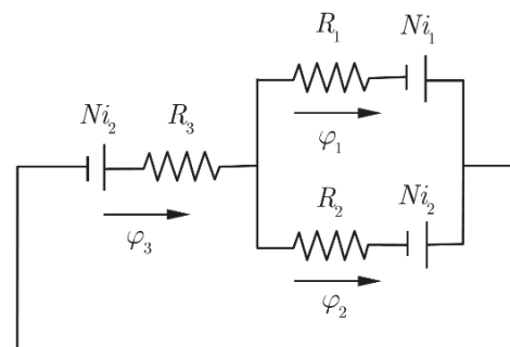
Fig. 3 Magnetic circuit of three-pole AMB [5]
