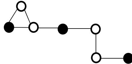
Fig. 5 MCDS
