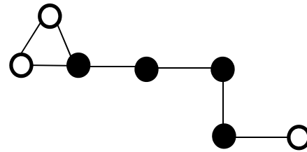
Fig. 4 IDS
