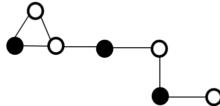
Fig. 6 CDS
