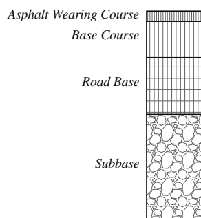
Fig. 1 Pavement superstructures
