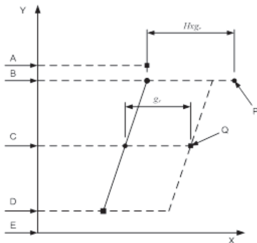
Fig. 1 Thermal Diagram [15]
