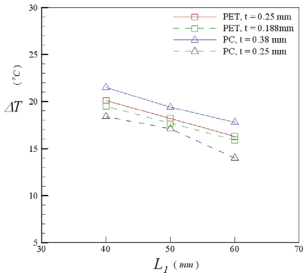
Fig. 13 \Delta T versus L_l . ( W_b = 60 mm)
