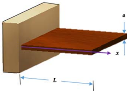
Fig. 1 Rectangular Fin
