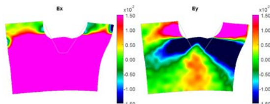
(d) Loading = 26.00kN
