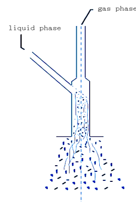
Fig. 2 Y type jet atomizer
