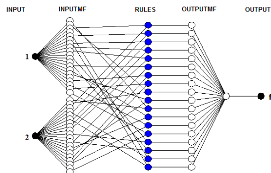
Fig. 3 ANFIS structure
