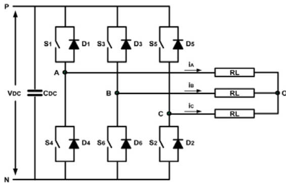
Fig. 3 2L-3P VSI
