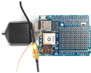
Fig. 7 Adafruit ultimate GPS data logger
