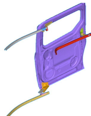
Fig. 2 Sliding door system
