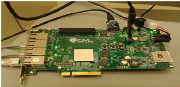
Fig. 6 NetFPGA-1G-CML
