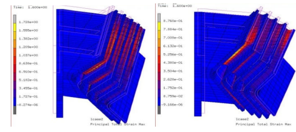
(c) Strain at longitudinal load (d) Stress at longitudinal load
