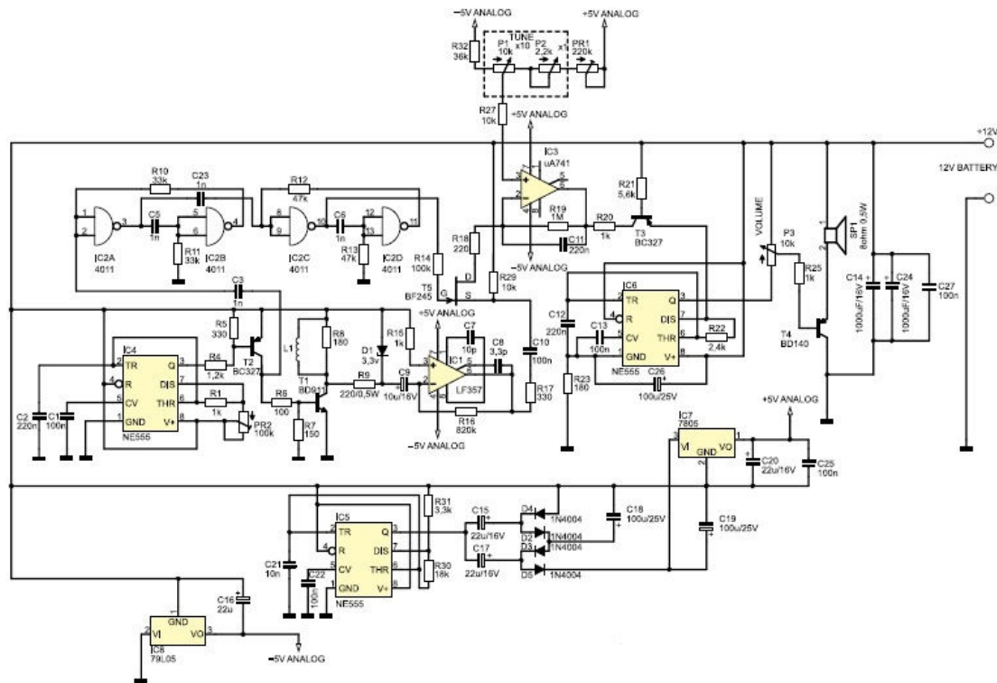
Fig. 10 Metal Detector
