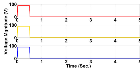
Fig. 4 (d) V_R, V_Y, V_B voltage magnitude during TLGF
