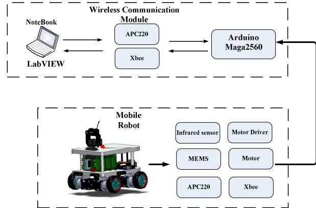
Fig. 3 Communication Module
