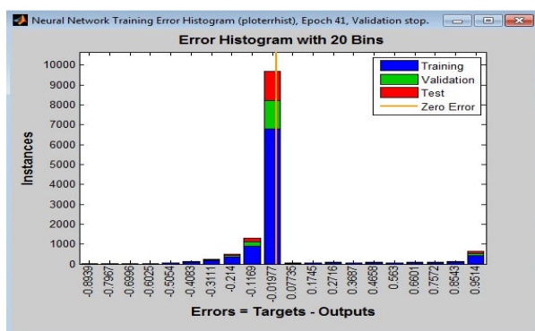
Fig. 7 Error Histogram
