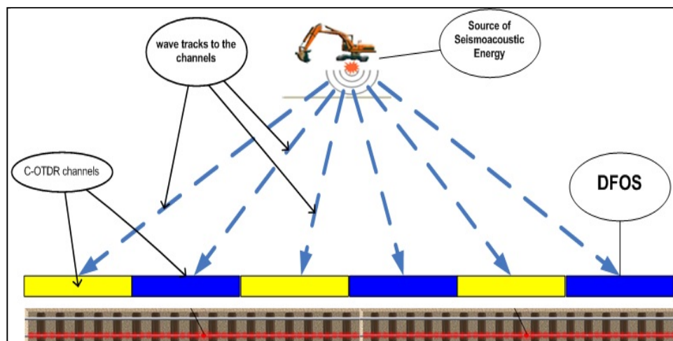
Fig. 1 C-OTDR Channels
