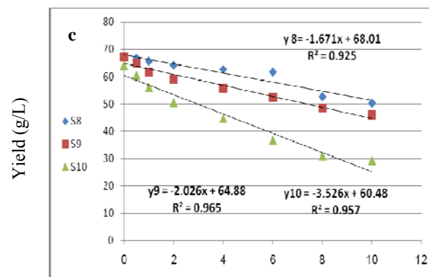
Fig. 4 (a) Effect of cadmium on yield of S. cerevisiae F-707, S. cerevisiae FA-91 and S. cerevisiae FF-725 strains; (b) Effect of cadmium on yield of S. cerevisiae F-235, S. cerevisiae F-25, S. cerevisiae FK-727, S. cerevisiae FK-727 and S. cerevisiae FC-620 strains; (c) Effect of cadmium on yield of S. cerevisiae FH-620, S. cerevisiae FAT-12 and S. cerevisiae F-514 strains
