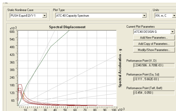
Fig. 17 (d) Model IIC (strut infill-Soft storey-ASCE/SEI 41), R=3.61
