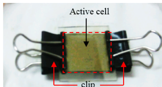
Fig. 4 DSSC prototype
