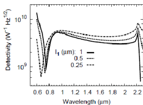
Fig. 7 Detection parameter of an n^+nn^+ diode
