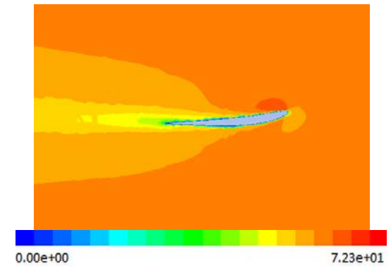
(d) Angle of attack = 6^{\circ}
