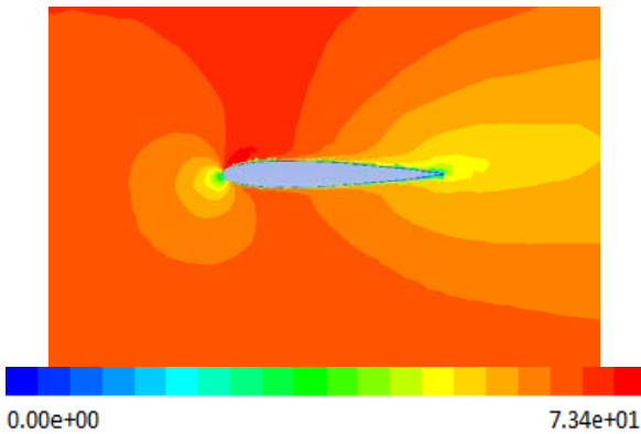
(d) Angle of attack = 6^\circ
