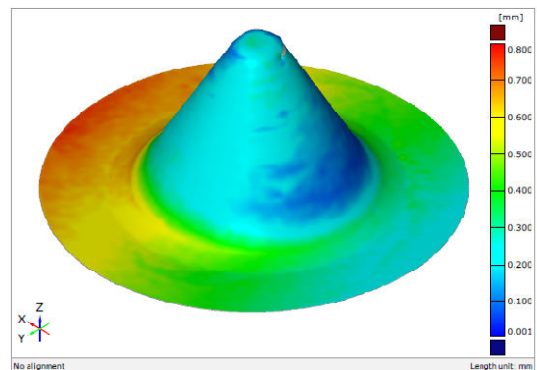
(b) SUS 304 thickness distribution
