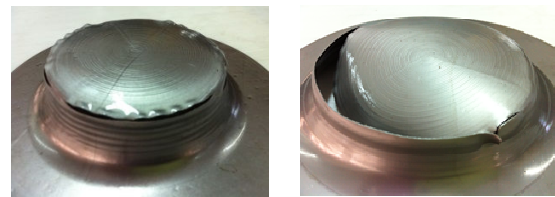
(a) SS 400 (b) SUS 304
